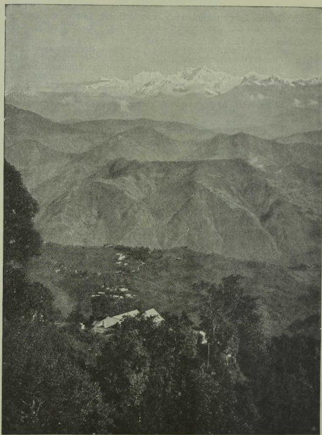
Ketten- (Zalen-) Bau des Himalaja, von Darjiling aus gesehen.
