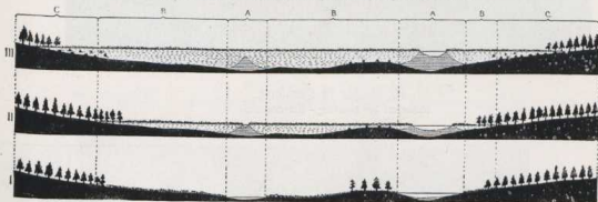
43. Moorbildung. Aus Braun, Das Ostseegebiet. Leipzig, B. G. Teubner.
