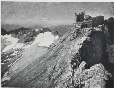
108. Zugspitze (Gipfel).
