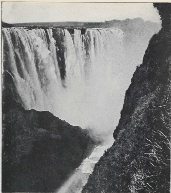
198. Die Vittoria- Fälle des Sambesi.
