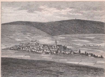
Fig. 22. Oberwiesenthal mit dem Fichtelberg.
