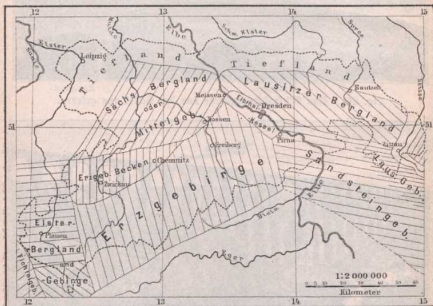
Fig. 23. Oberflächenformen und Hauptflüsse Sachsens. (Vergl. Penck, Unser Wissen von der Erde, II.)
