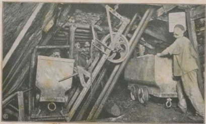
Füllort und Hauptschachtanschlagspunkt unter Tage.
