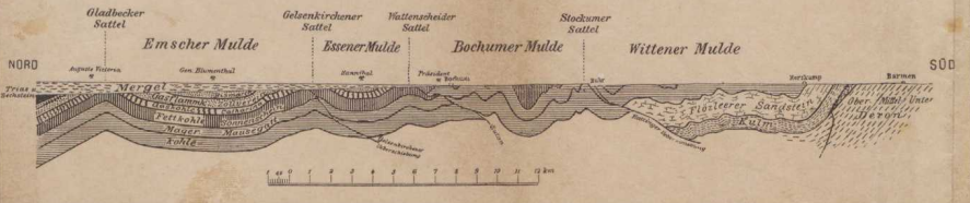
Schematisches Querprofil durch das Ruhrbecken.
